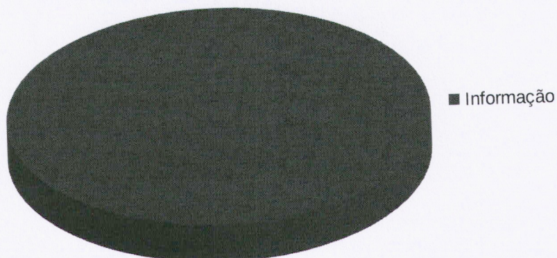
Gráfico 4 - Característica Manifestações
