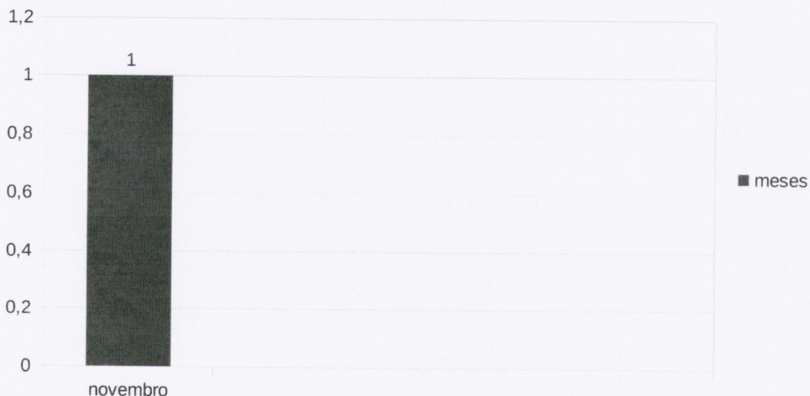
Gráfico 1 - Manifestações Registradas
